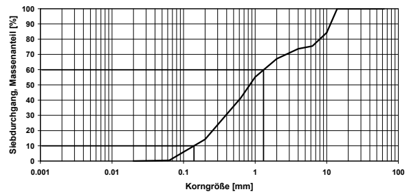
Korngrößenverteilung Brunnen 1 - BP 9
