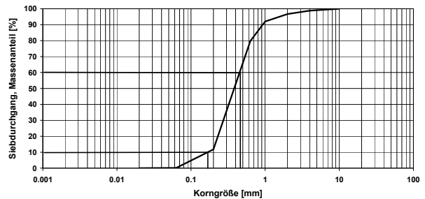
Korngrößenverteilung Brunnen 1 - BP 6
