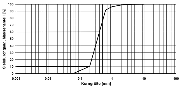
Korngrößenverteilung Brunnen 1 - BP 7
