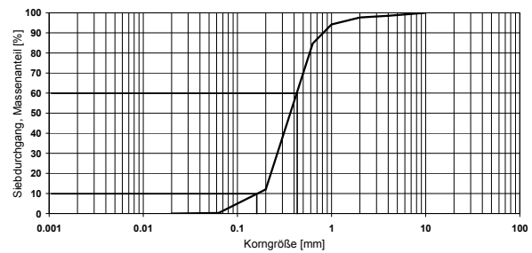
Korngrößenverteilung MS-05 - BP 8
