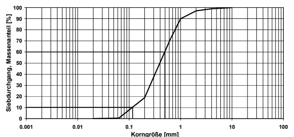
Korngrößenverteilung Brunnen 1 - BP 10
