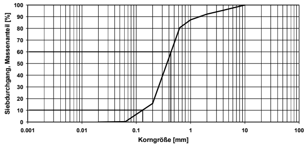
Korngrößenverteilung Brunnen 1 - BP 5
