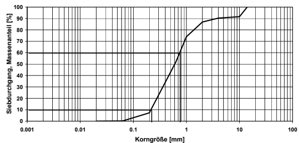
Korngrößenverteilung Brunnen 1 - BP 11
