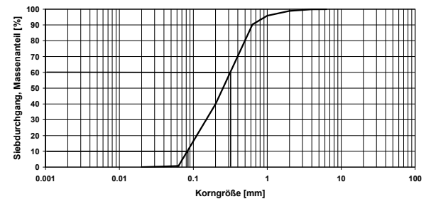
Korngrößenverteilung Brunnen 1 - BP 8
